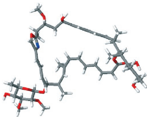
Figure 3. Calculated structure of chivosazole A (1).
