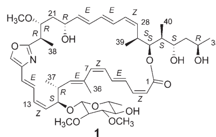
Figure 4. Absolute configuration of chivosazole A ( 1 ).
